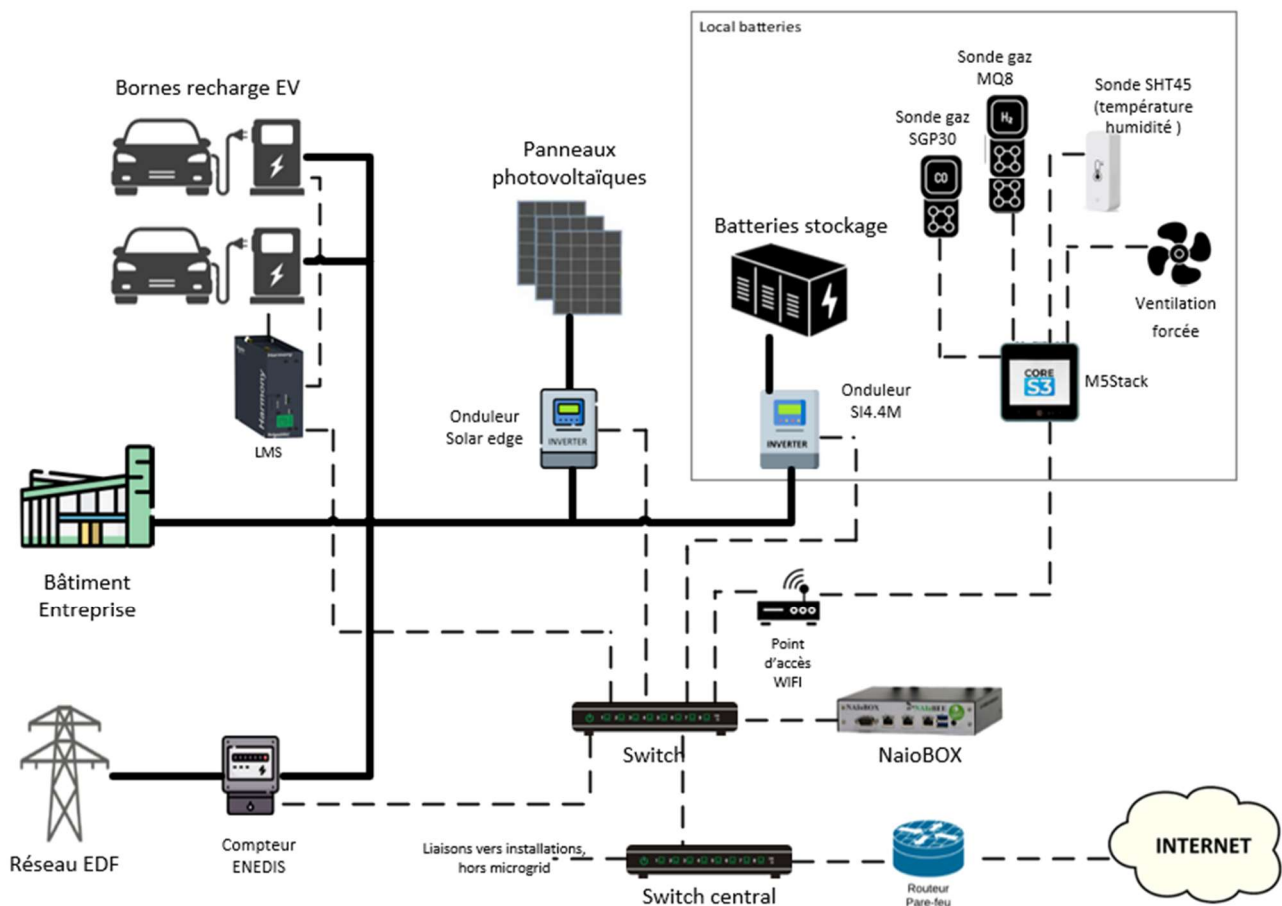
Figure 1 : Microgrid supervisé par Naiobox
