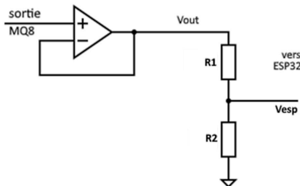
Figure A2 : Circuit d'adaptation de tension pour ESP32
