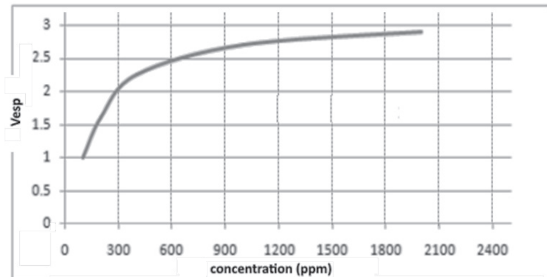
Figure A4 : Tension CAN ESP32 en fonction de la concentration en H2
