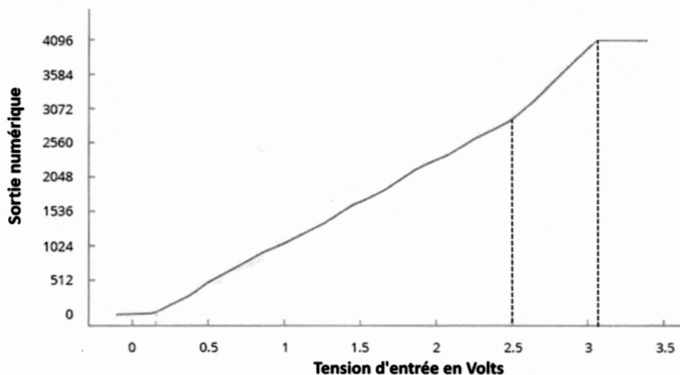
Figure A5 : Caractéristique CAN ESP32
